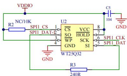
外置FLASH电路
