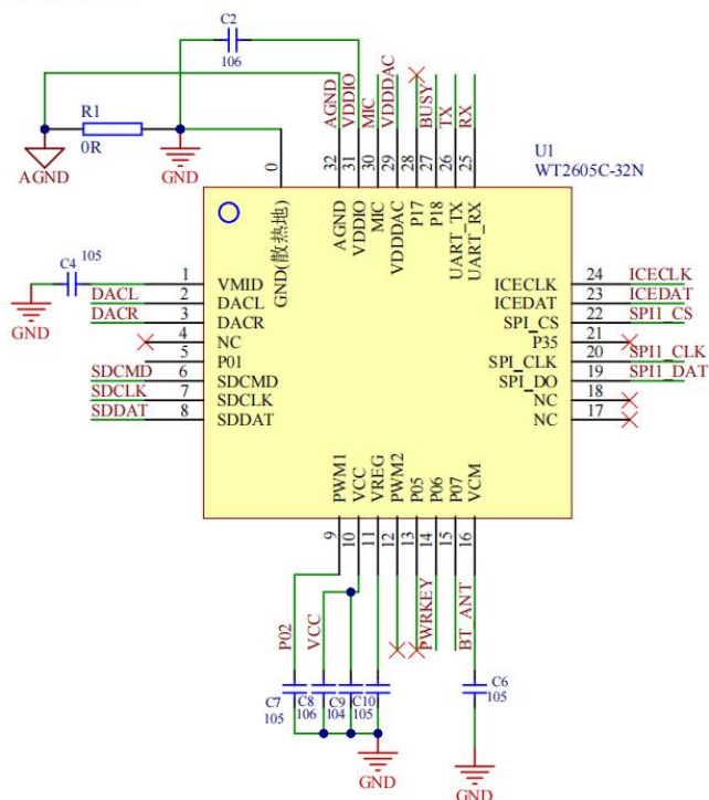
语音芯片
